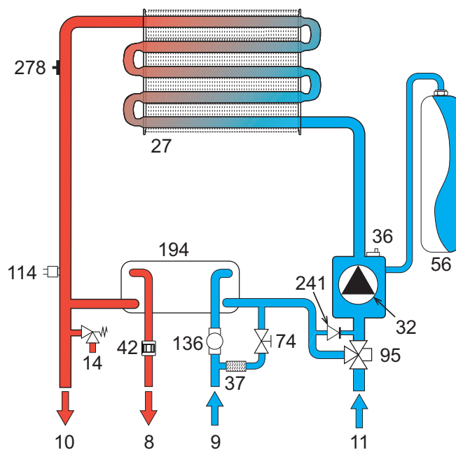
рис. 22- Контур отопления
