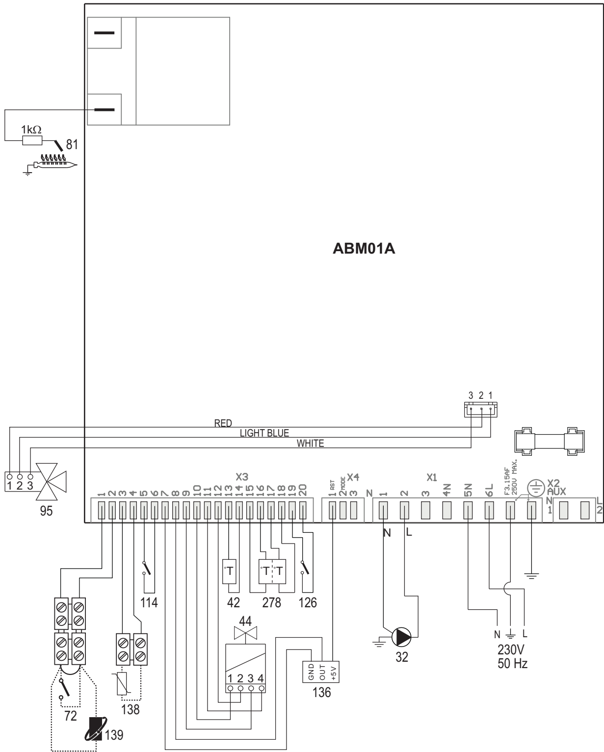
рис. 23- Электрическая схема
