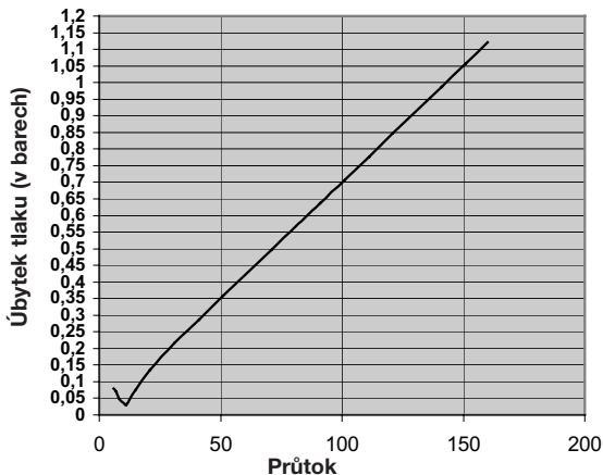
Úbytek tlaku
