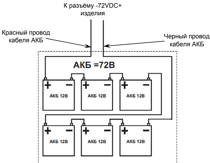
Рисунок 7 — схема монтажа аккумуляторной батареи.
