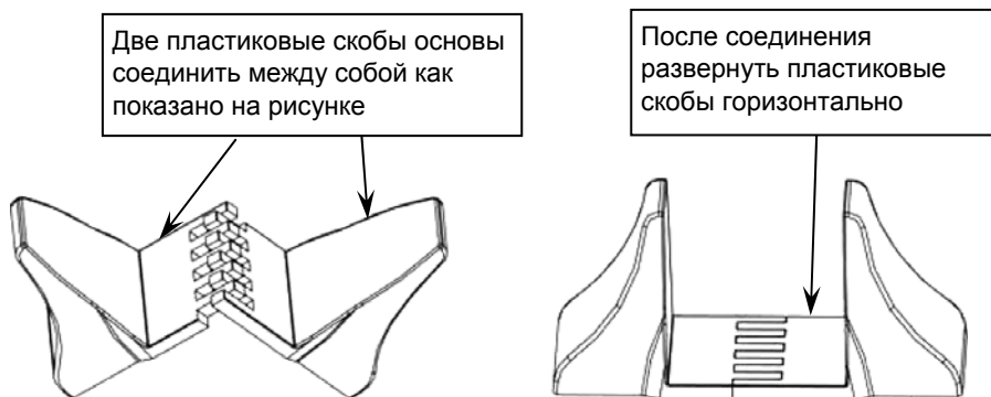
Рисунок 5 - сборка пластиковых основ для вертикальной установки изделия
