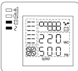
Рисунок 10 — состояние ЖК-дисплея и индикаторов и режиме «РЕЗЕРВ»
