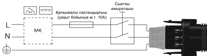
19-сур. ALPNA текерімен қосылым мысалы, 1 x 230 В ±10 %, 50/60 Гц, қорғанышты жерге тұйықтау
