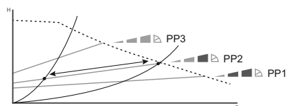
24-сур. Пропорционалды реттеудің үш қисығы/баптаулары
