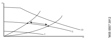
Рис. 26 Настройки трех кривых при фиксированной частоте вращения
